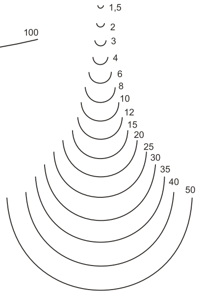
VPICH SWEEP 10
